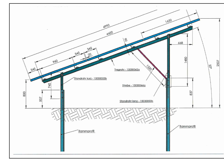
Schnitt Photovoltaik-Anlage M 1:50
